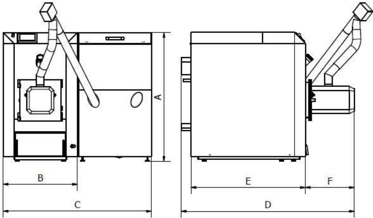
Parametry techniczne Rysunek nr 3. Wymiary instalacyjne kotłów
